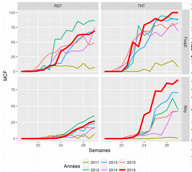
Evolution des attaques de mildiou sur le réseau régional de surveillance : Comparaison des fréquences de ceps atteints (MCF) sur parcelles références (REF) et témoins (TNT)
